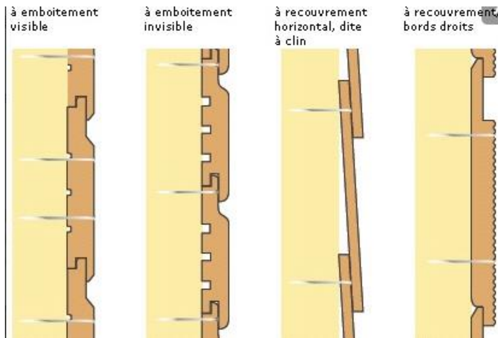
Différentes poses de bardage La pose retenue est à emboîtement visible, vis apparente
